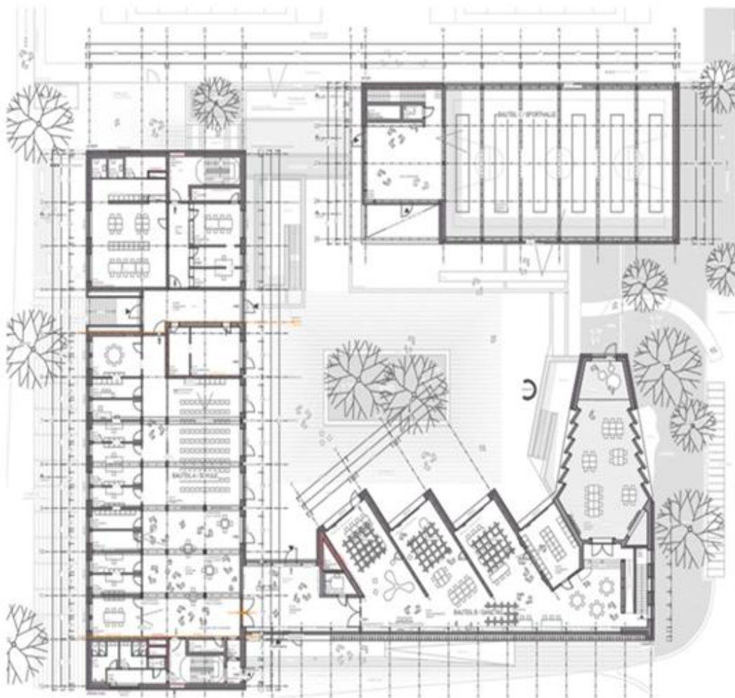
Entwurfsplanung – Grundriss Erdgeschoss
