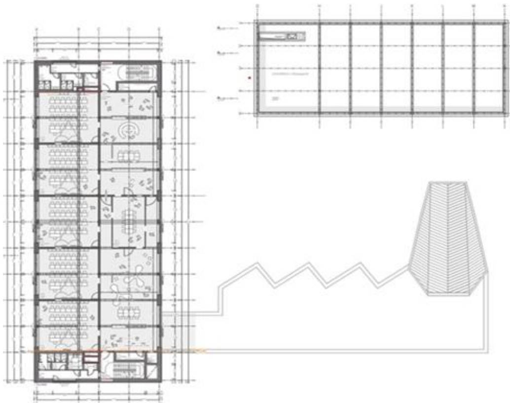
Entwurfsplanung – Grundriss 1. Obergeschoss
