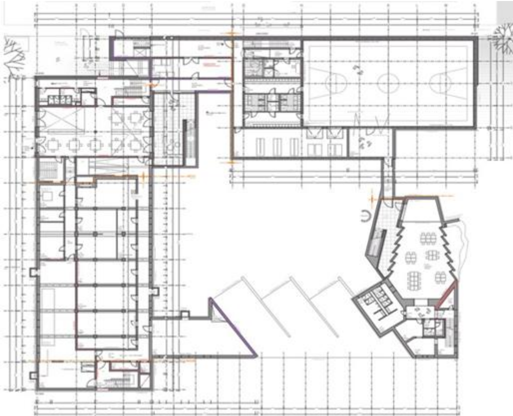
Entwurfsplanung – Grundriss Untergeschoss
